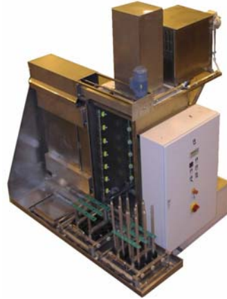
Sonderanlage zur Außen- und Innenreinigung von Rohren
